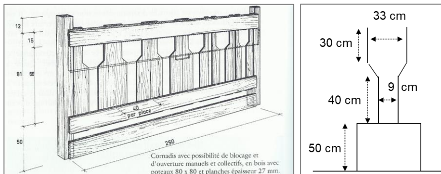
Fig. 2. Esempio di cattura in legno e relative misure complessive e per singola unità (Fonte: Institut de l'élevage)
